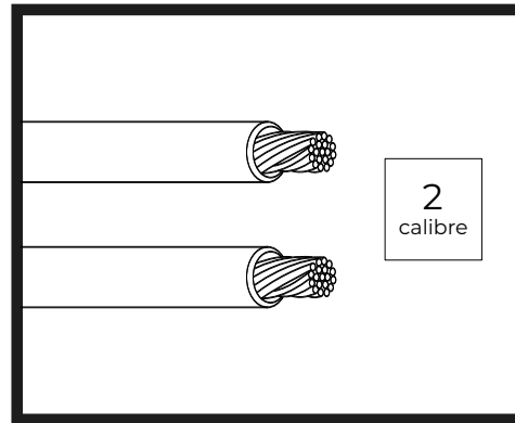
Dos líneas calientes de 120V en cable #2 THHN de cobre
