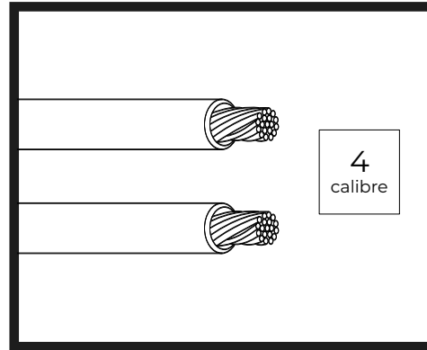
Dos líneas calientes de 120V en cable #4 THHN de cobre
